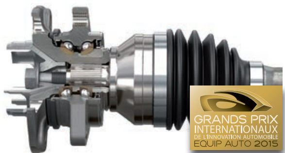
ПРЕССО-ШЛИЦЕВОЕ СОЕДИНЕНИЕ
