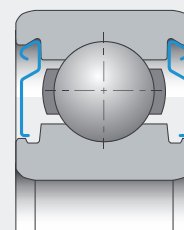
BLINDAGEM POR DEFLETORES (ZZ suffixo)
