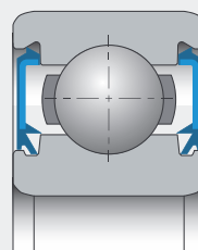
VEDAÇÃO DE CONTATO DUPLO (EE suffixo)
