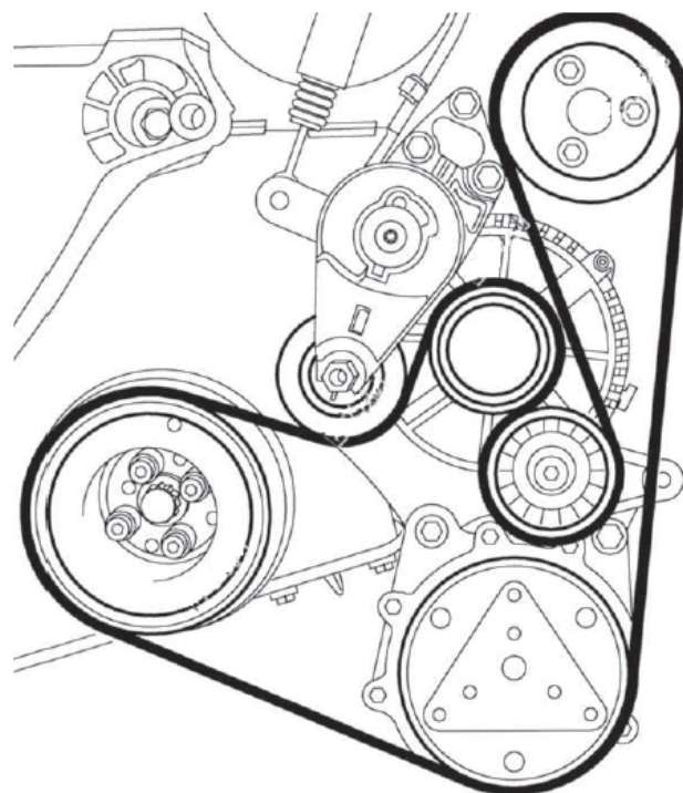
Fijación del rodillo de reenvío (Ref. NTN-SNR GA357.06) de la correa (únicamente para los vehículos con aire acondicionado)
