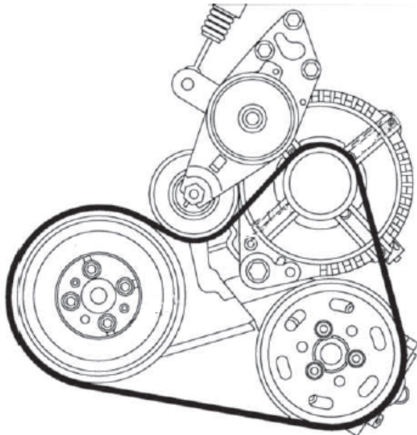
Recorrido de la correa de accesorios (vehículo sin aire acondicionado)
