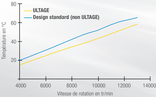
Températures de fonctionnement
