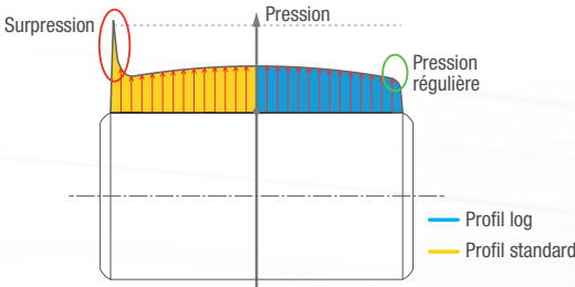
Pressions de contact sur chemin
