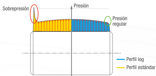
Presiones de contacto sobre la pista
