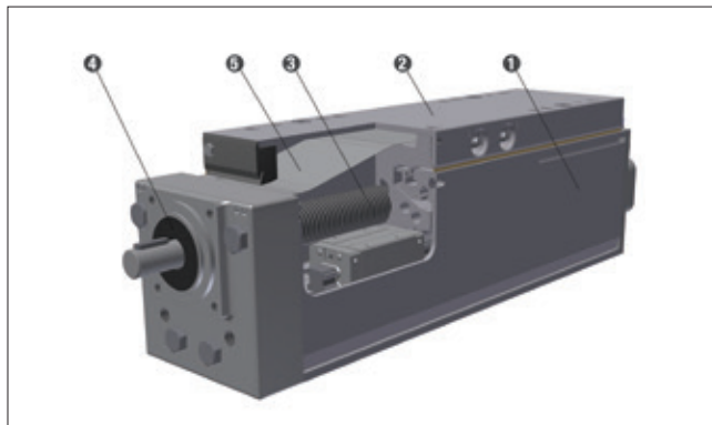
Bild 1.2 ____ Aufbau Spindelachse
