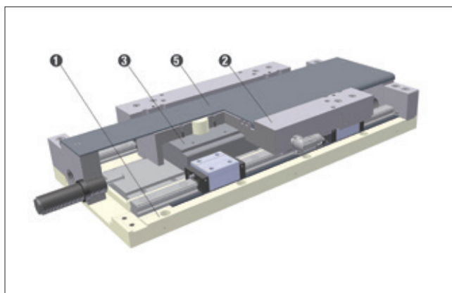
Bild 1.4 ____ Aufbau Linearmotorachse
