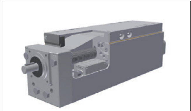
Bild 5.5 ____ AXF mit Spindeltrieb
