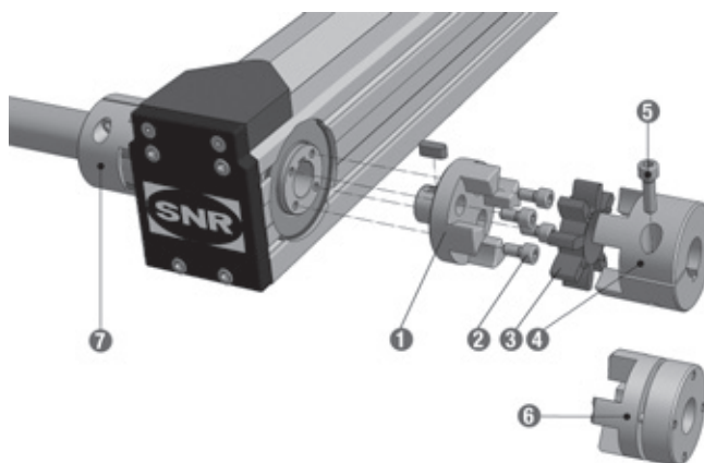
Bild 3.9 _____ Kupplungsmontage an Linearachsen mit Zahnriementrieb
