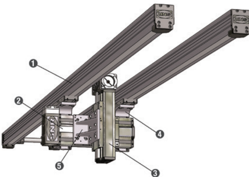
Bild 7.5 ____ Dreiachssystem AXC_Z – AXDL_Z - AXDL_Z
