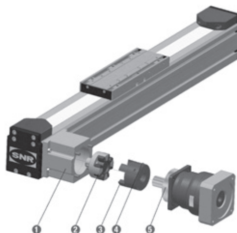
Bild 3.10 ____ Motormontage an Linearachsen mit Zahnriemenantrieb und Kupplungsglocke
