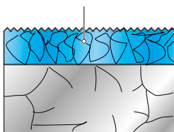
Fig. 11: Sección de una jaula de chapa de acero con tratamiento de fosfatación
