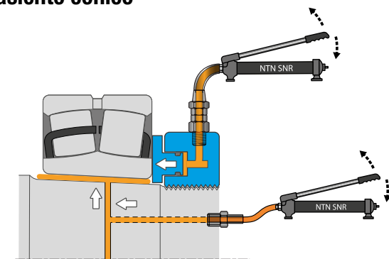
Uso simultáneo de la tuerca hidráulica asociada a la inyección de la película de aceite
