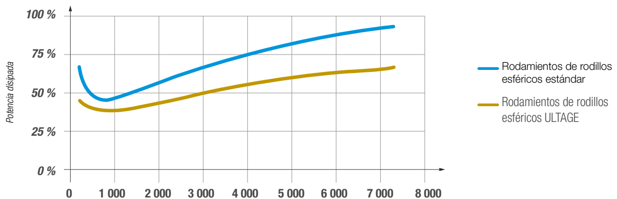
Fig. 2: comparativa de la potencia disipada en función de la velocidad.
