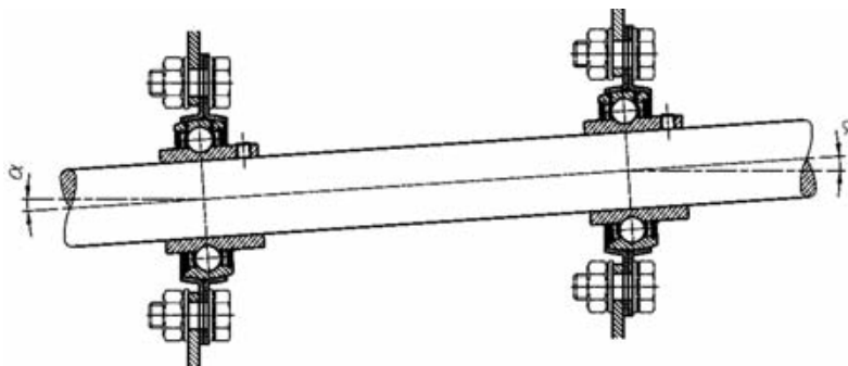
Soportes de chapa de acero \alpha = \pm 5^\circ
