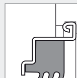
Уплотнение L3
