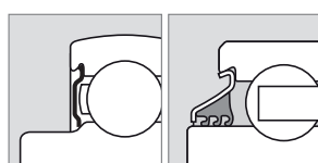
Уплотнение А
