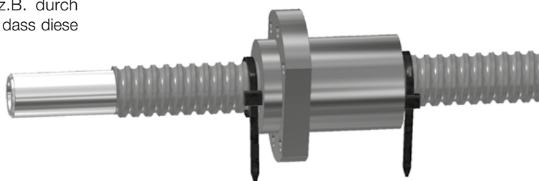
Bild 3.2 _____ Sicherung von Kugelgewindemuttern
