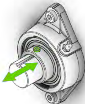
Remplazando los tornillos de fijación, los rodamientos insertos del tipo UC y US se pueden utilizar con soportes flotantes.
