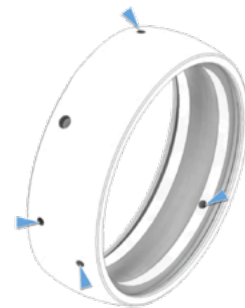
Sistema G2: Anillo exterior con cuatro orificios de lubricación en dos planos
