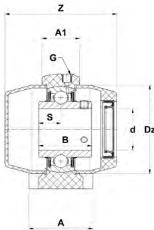
MUCPPL + Tapas protectoras
