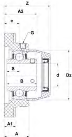
MUCFPL + Tapas protectoras
