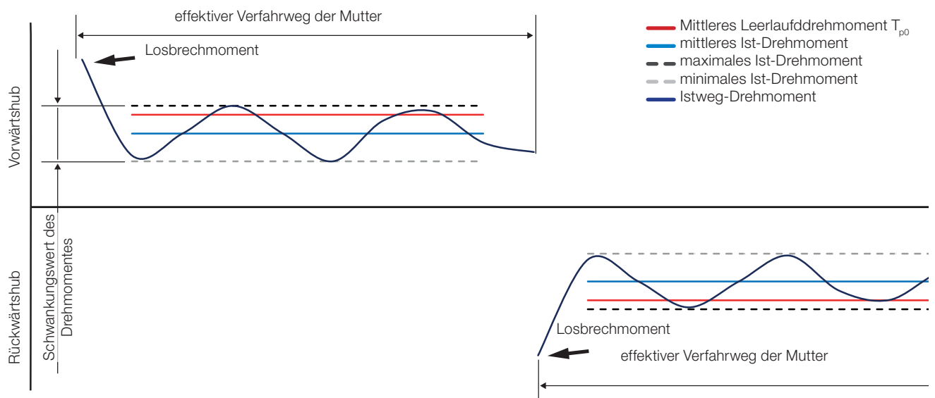
Bild 2.11 ____ Leerlaufdrehmomentschwankung von Kugelgewindetrieben
