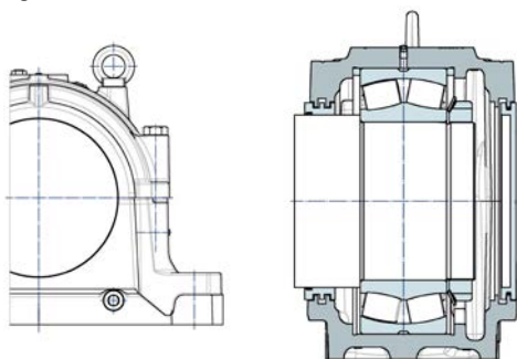
B. Montage avec roulement en extrémité d'arbre
