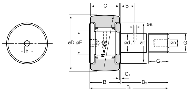
KR -- H (avec cage)
