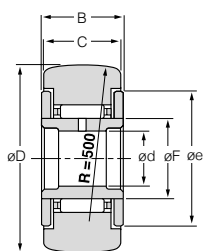
NATR (avec cage)
