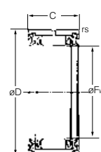
RNA49 -- LL (avec étanchéité des deux côtés)
