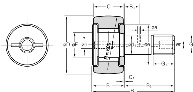
KRV (avec étanchéité sans cage)
