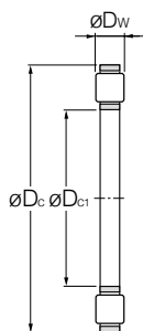
K811, K812 Cage à rouleaux
