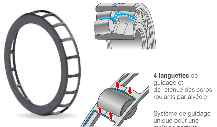
EA – Cage en tôle d'acier emboutie
