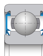
Étanchéités (avec contact) (« -EE »)
