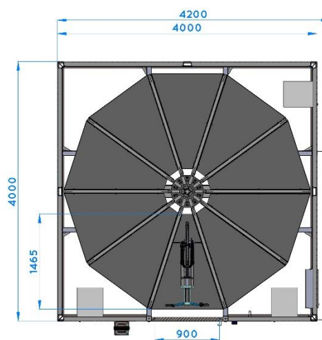
Détails de l'espace parking (unité : mm)
