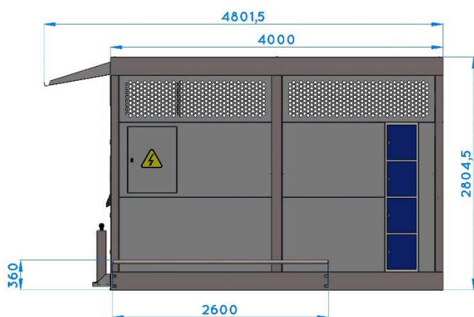
Vue de côté (unité : mm)
